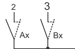
2x NO/NC contacts
