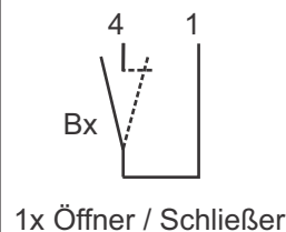
Anschlussbild M12 4Pol (02)
