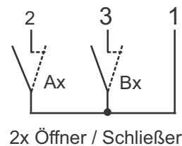
M12 5Pol (08)
